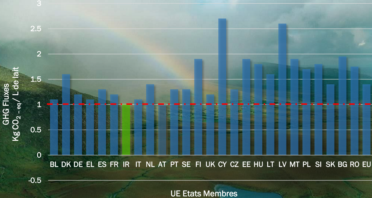
Emissions GES CHEPTEL LAITIER UE
