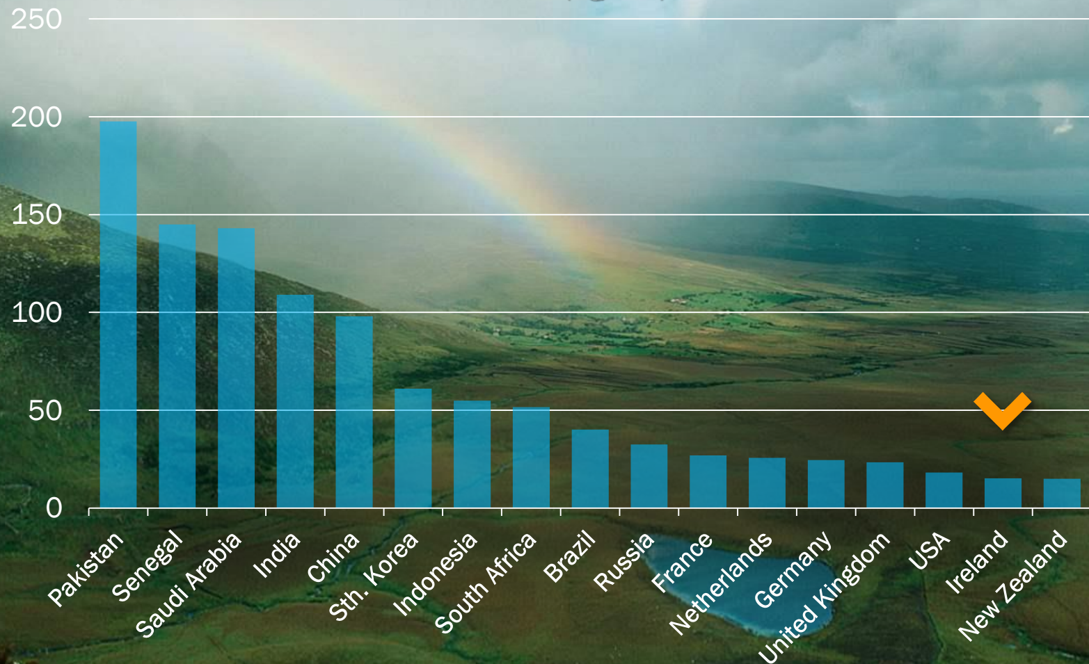
Pollution Atmosphérique Urbaine Moyenne annuelle PM10 (ug/m3)
